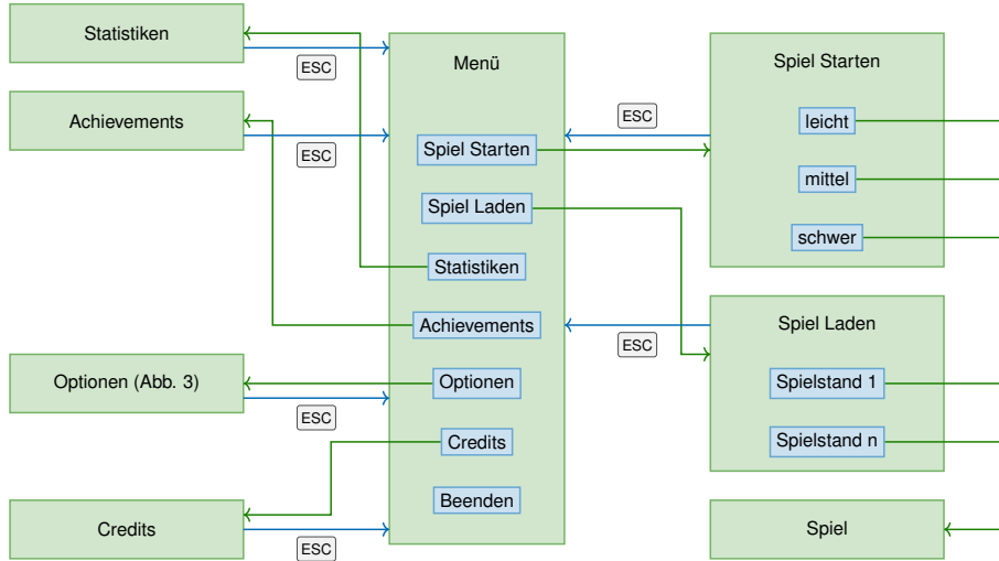
Abbildung 2: Die Menüstruktur von Irrgärten. Menüs werden als grüne Boxen, einzelne Schaltflächen als ...
